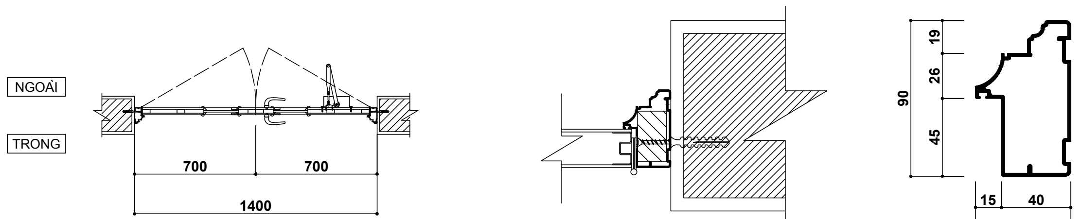
MẶT BẰNG
