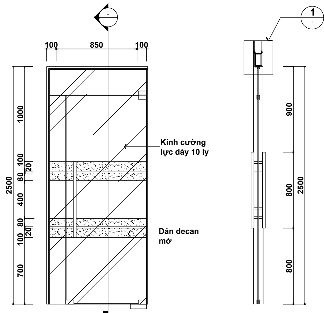
MẶT ĐỨNG
