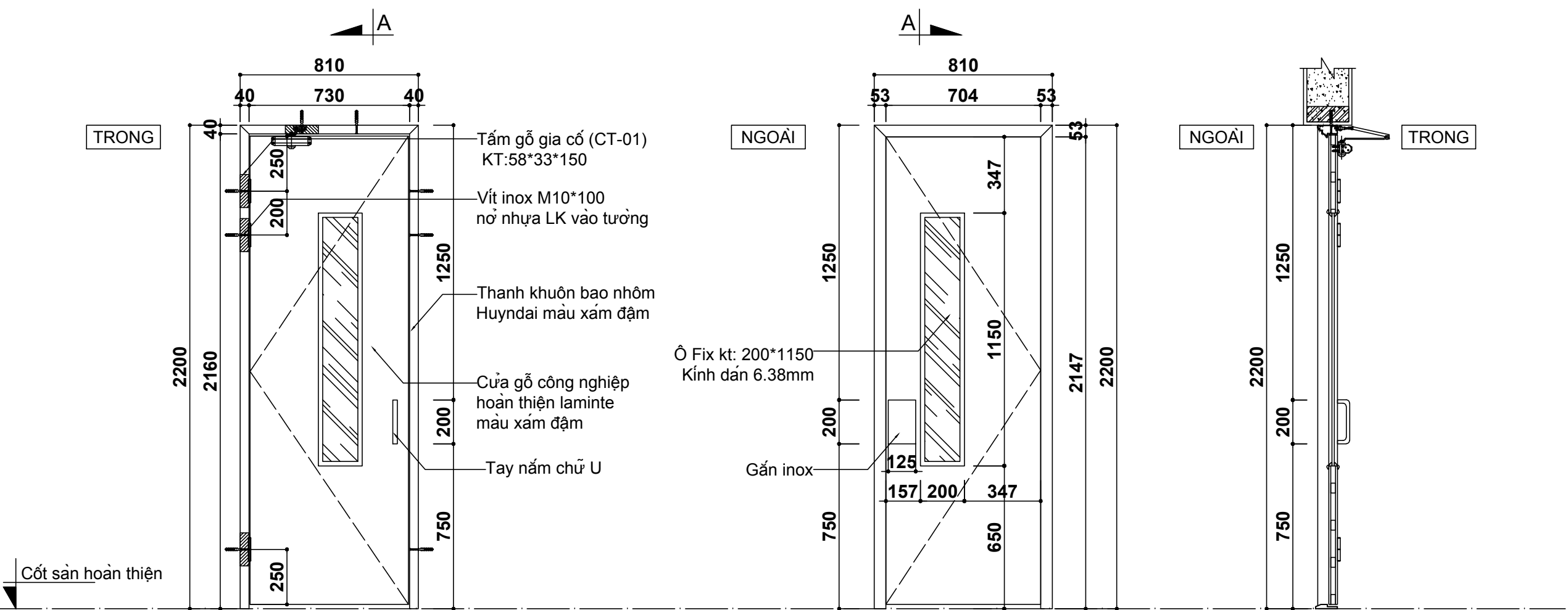
MẶT ĐỨNG
