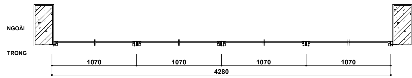
MẶT BẰNG
