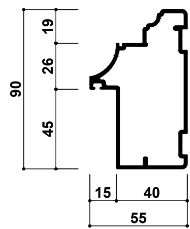
MẶT BÊN
