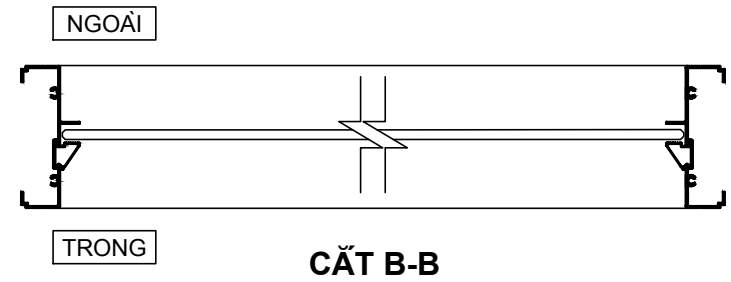
MẶT CẮT
