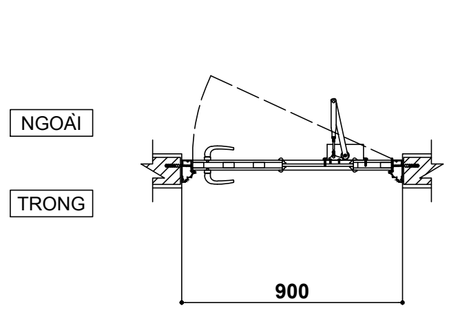
MẶT BẰNG
