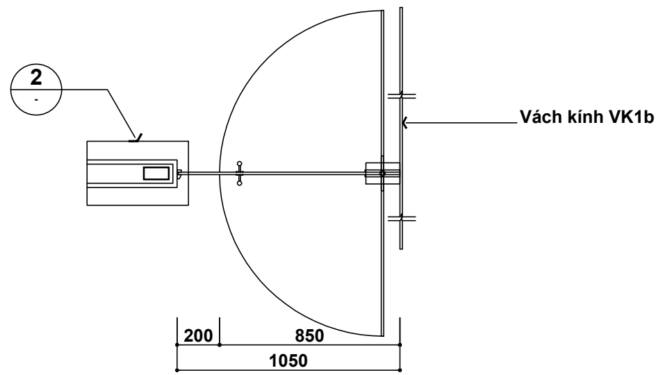
MẶT BẰNG
