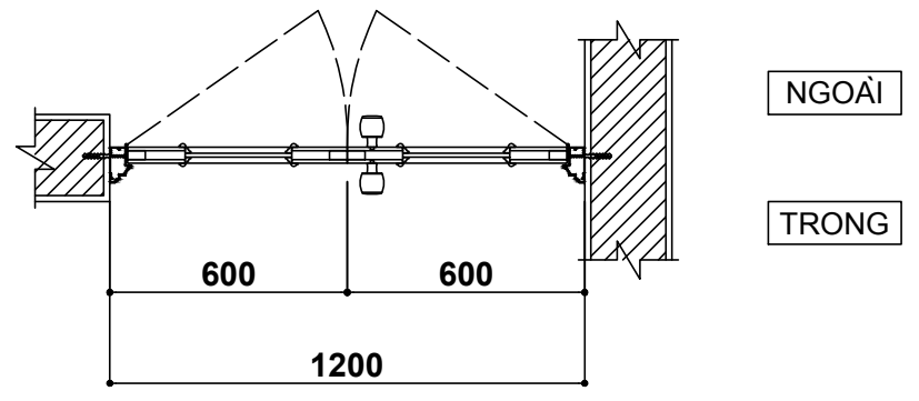
MẶT BẰNG
