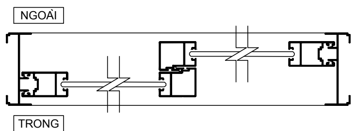
CẮT C-C
