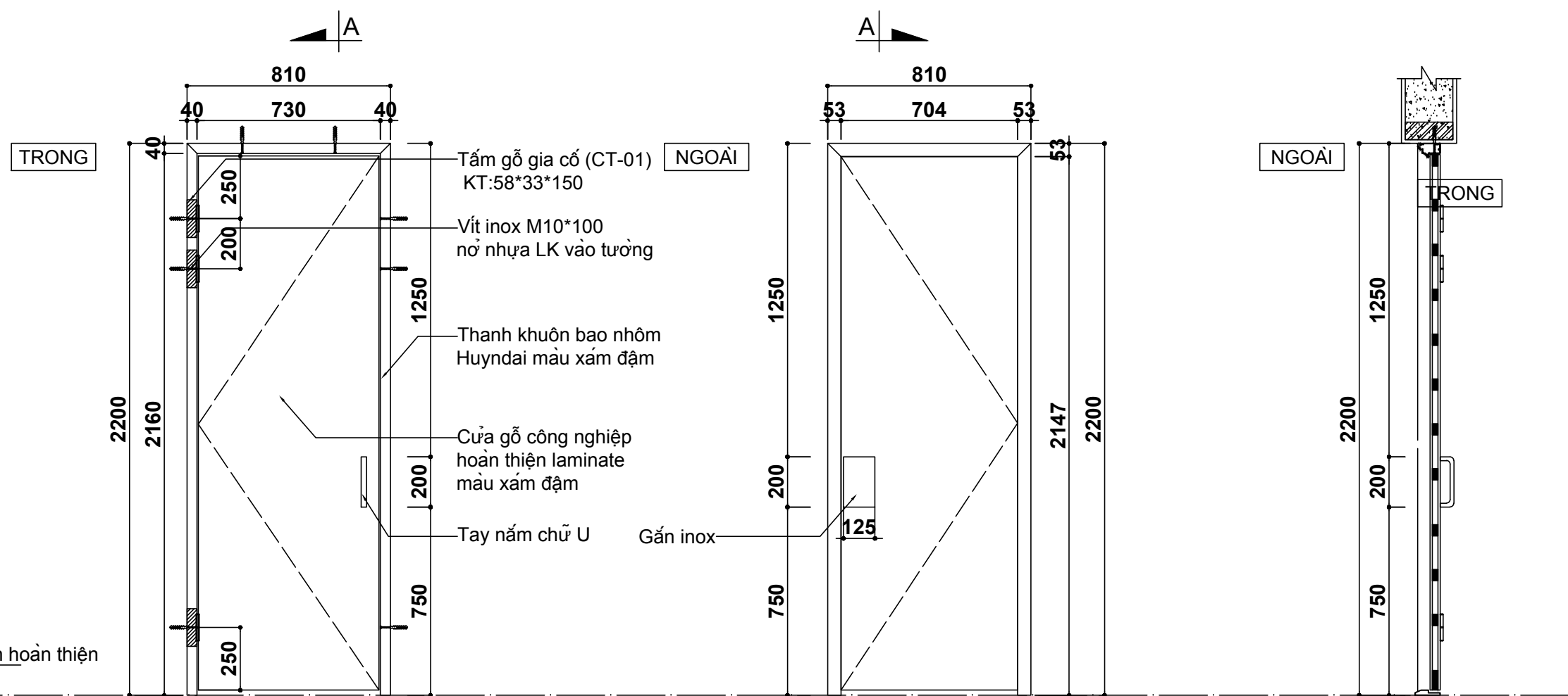
MẶT ĐỨNG
