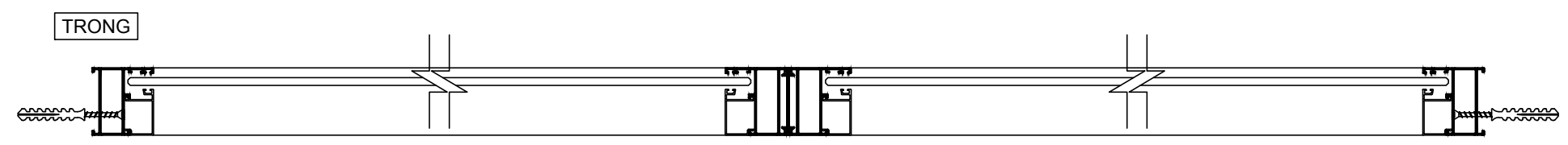
CẮT C-C
