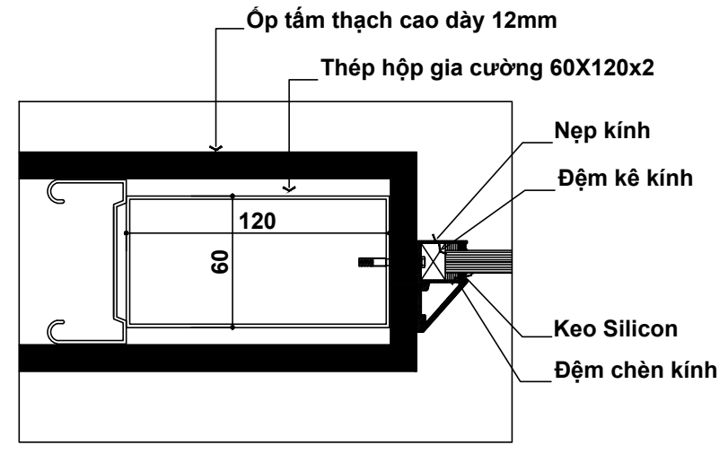
CHI TIẾT 2
