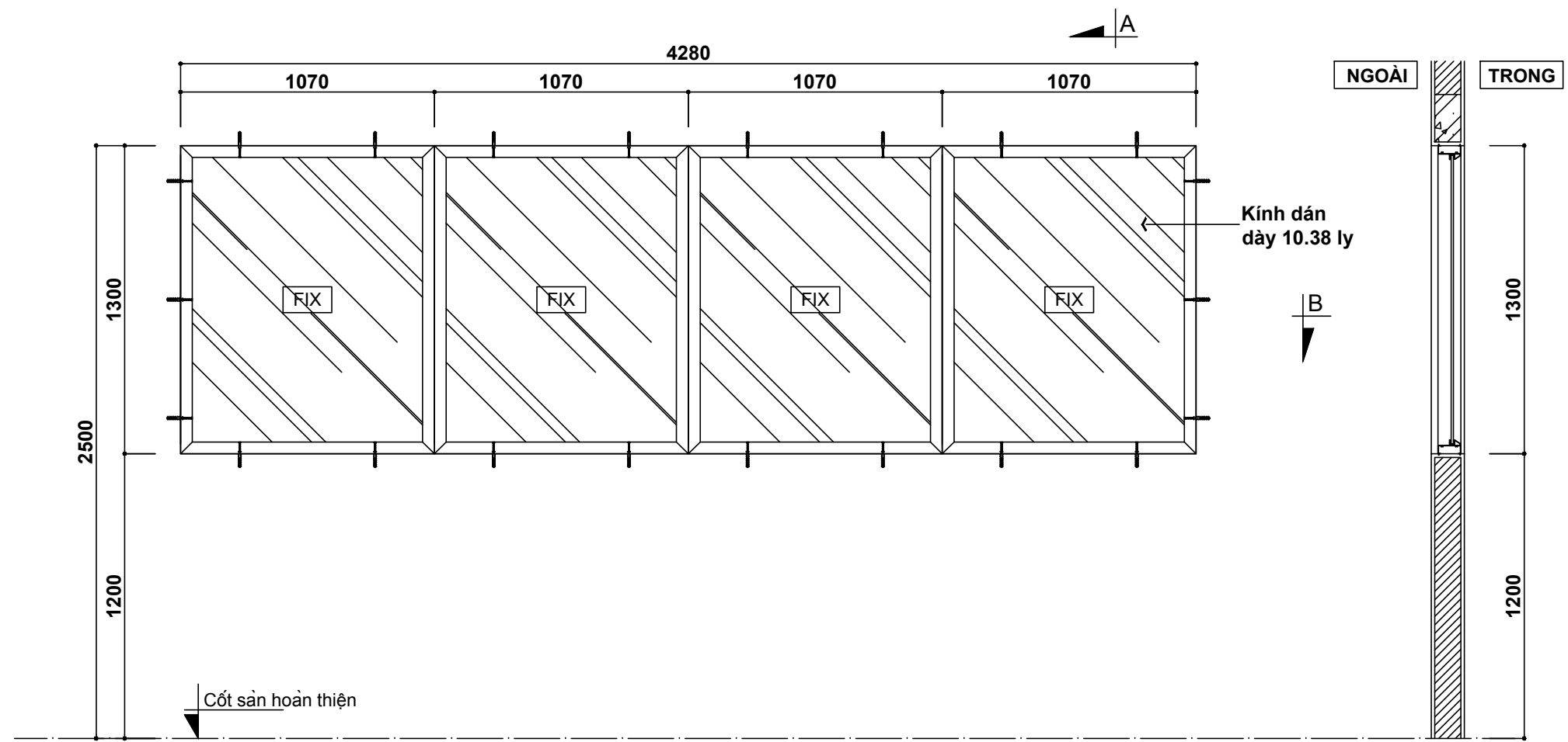
MẶT ĐỨNG
