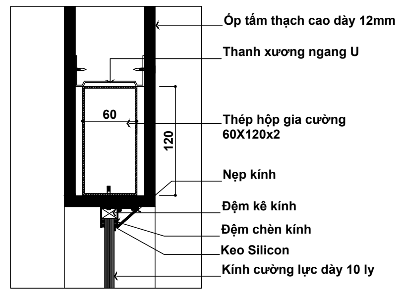
CHI TIẾT 1
