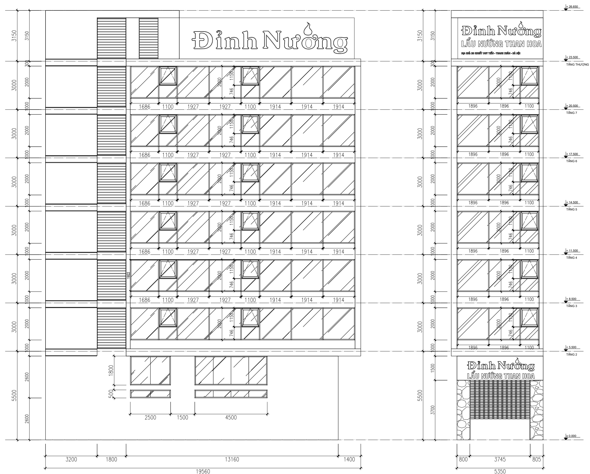
MẶT BÊN NHÀ TỈ LỆ: 1/80
